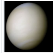
Venus
